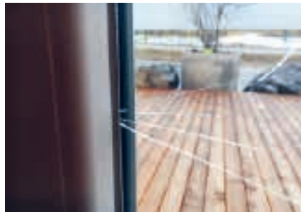
Thermischer Glasbruch
